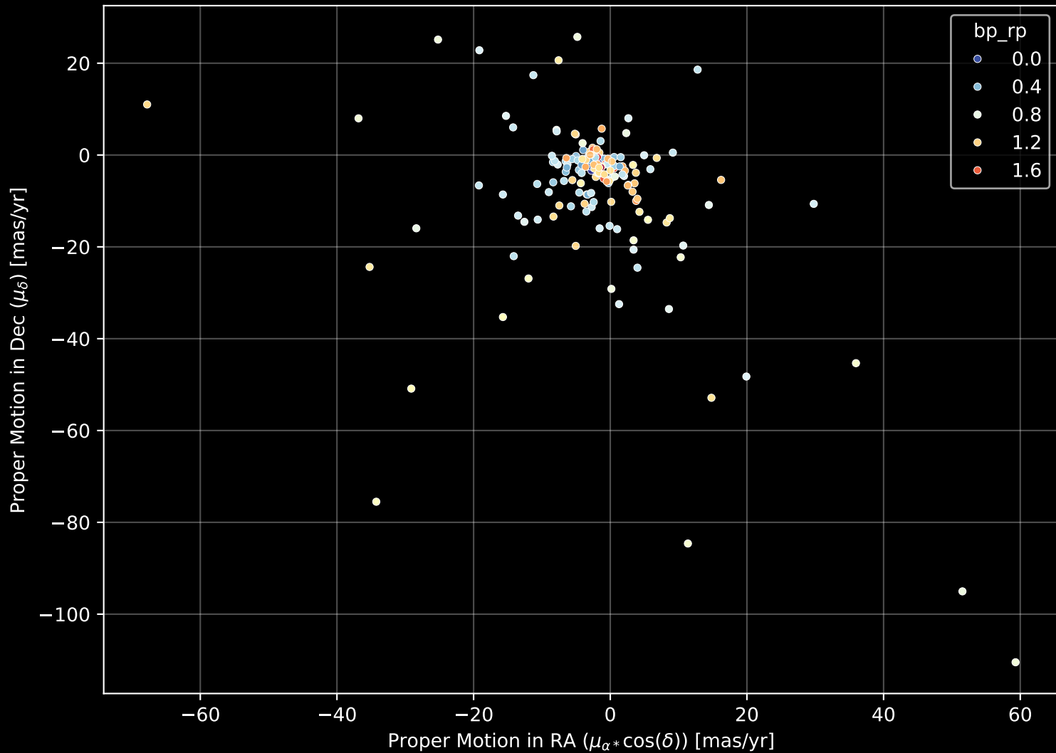
GALAH DR4 Field: [4120] Proper Motion Diagram (n= 171)
