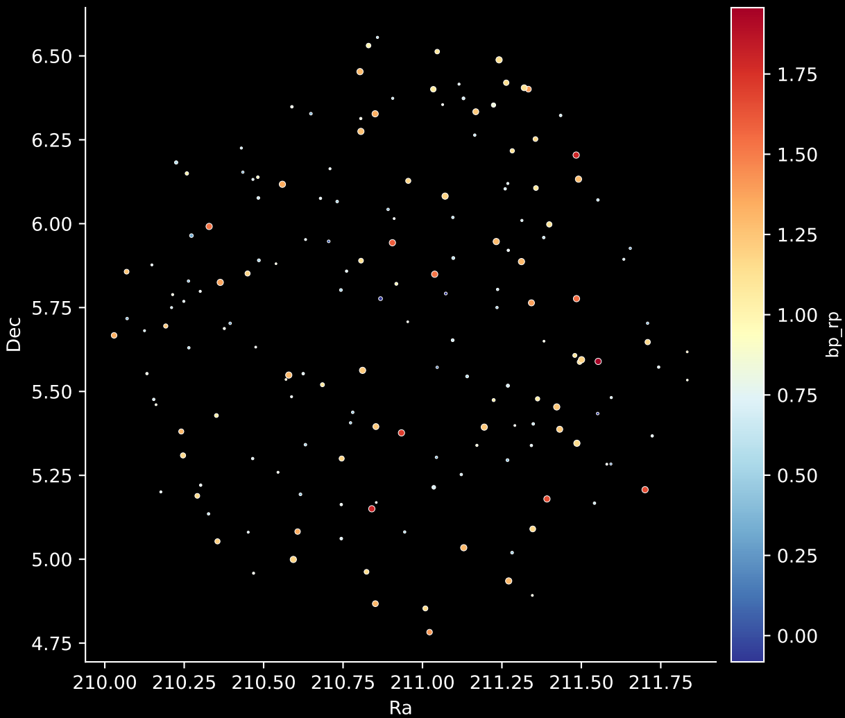
GALAH DR4 Field: [4120] Stars: 171
