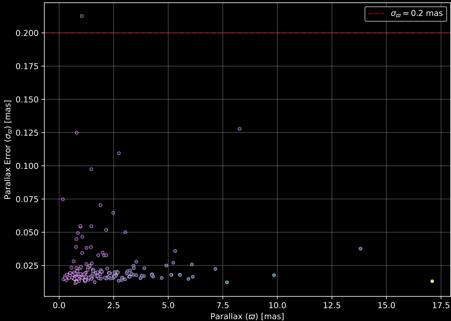
GALAH DR4 Field: [4120] Parallax Quality (n= 171)
