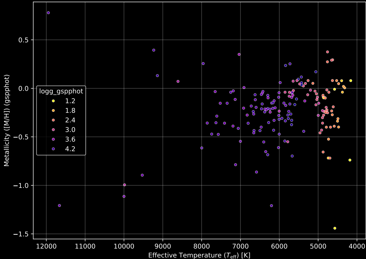
GALAH DR4 Field: [4120] Stellar Population Parameters (n= 171)
